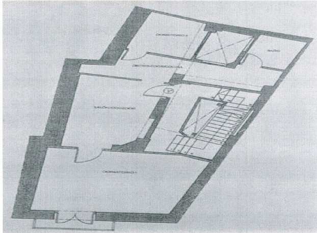
PLANTA TERCERA
